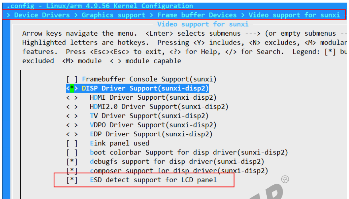
图 5-10: menuconfig
