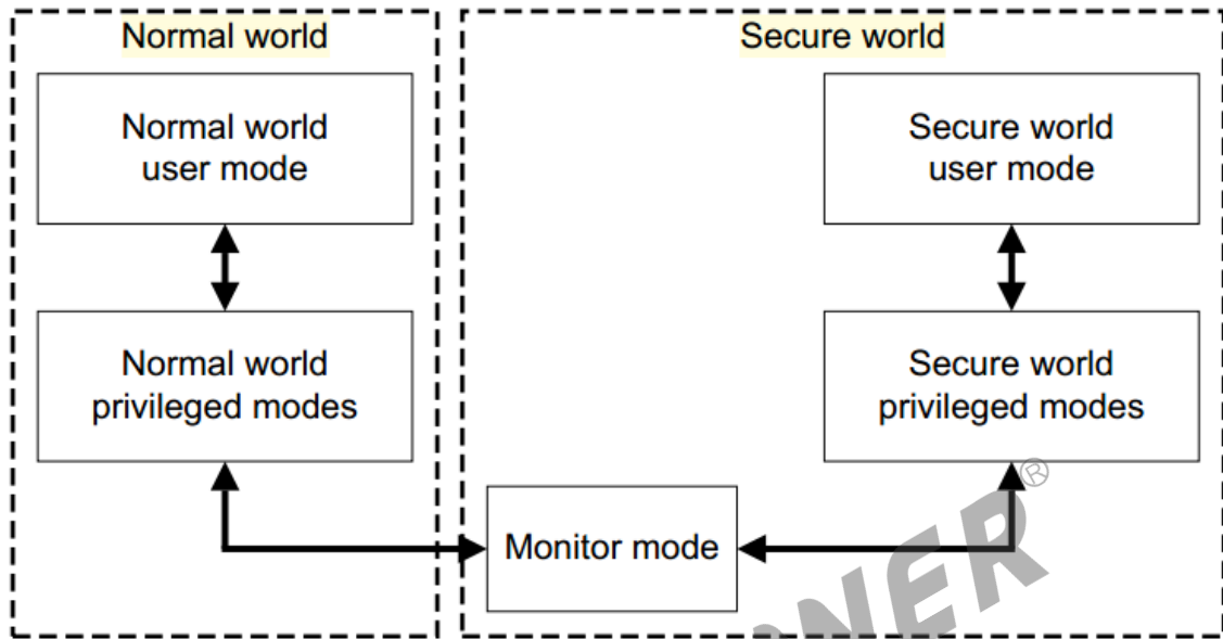
图 2-7: TrustZone 系统模型
