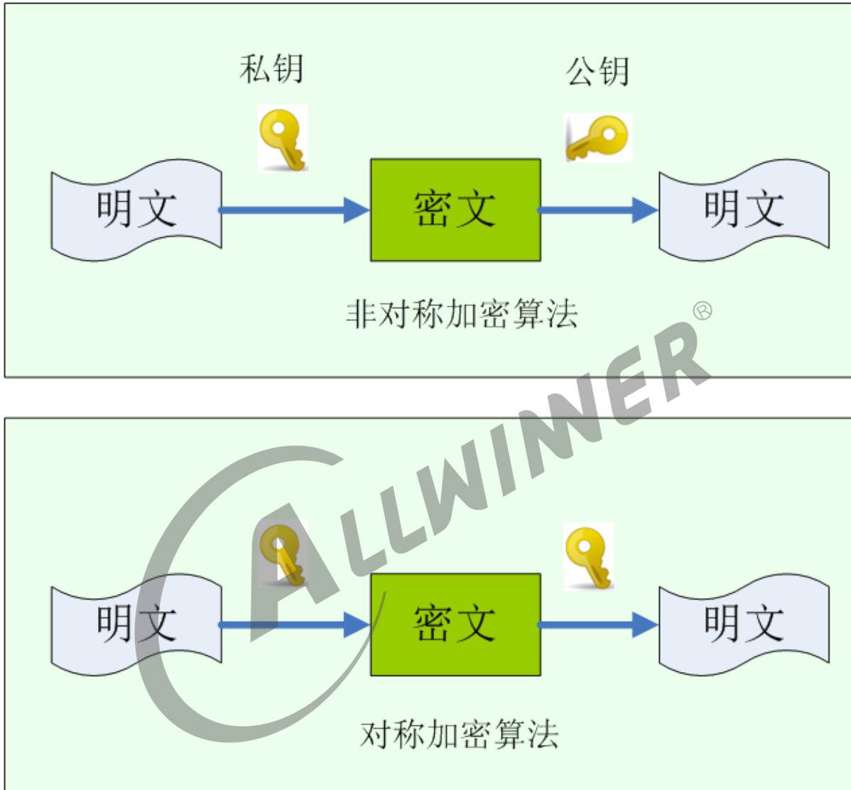
图 2-2: 对称及非对称加密
