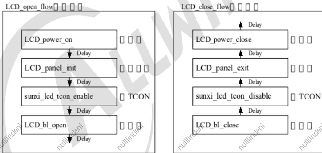
图 9: 开关屏流程
