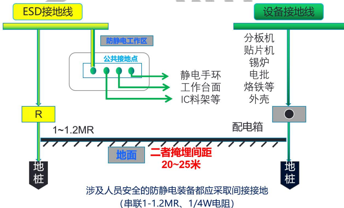
图 3-1 接地图示
