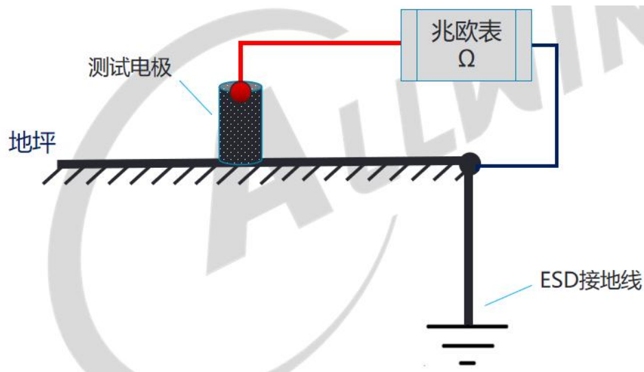
图 3-2 地坪接地
