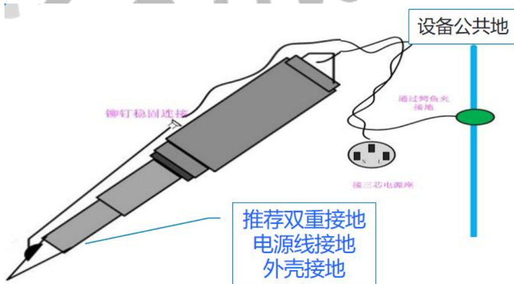
图 3-7 烙铁接地
