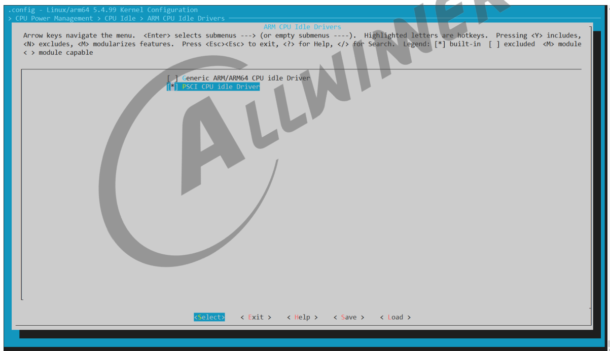
图 2-1: cpuidle 配置-2
