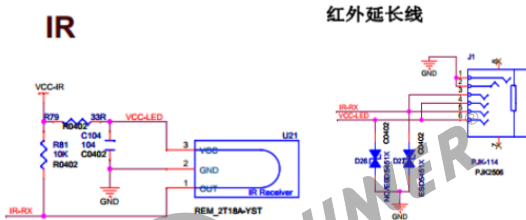
图 2-1: IR-RX 模块
