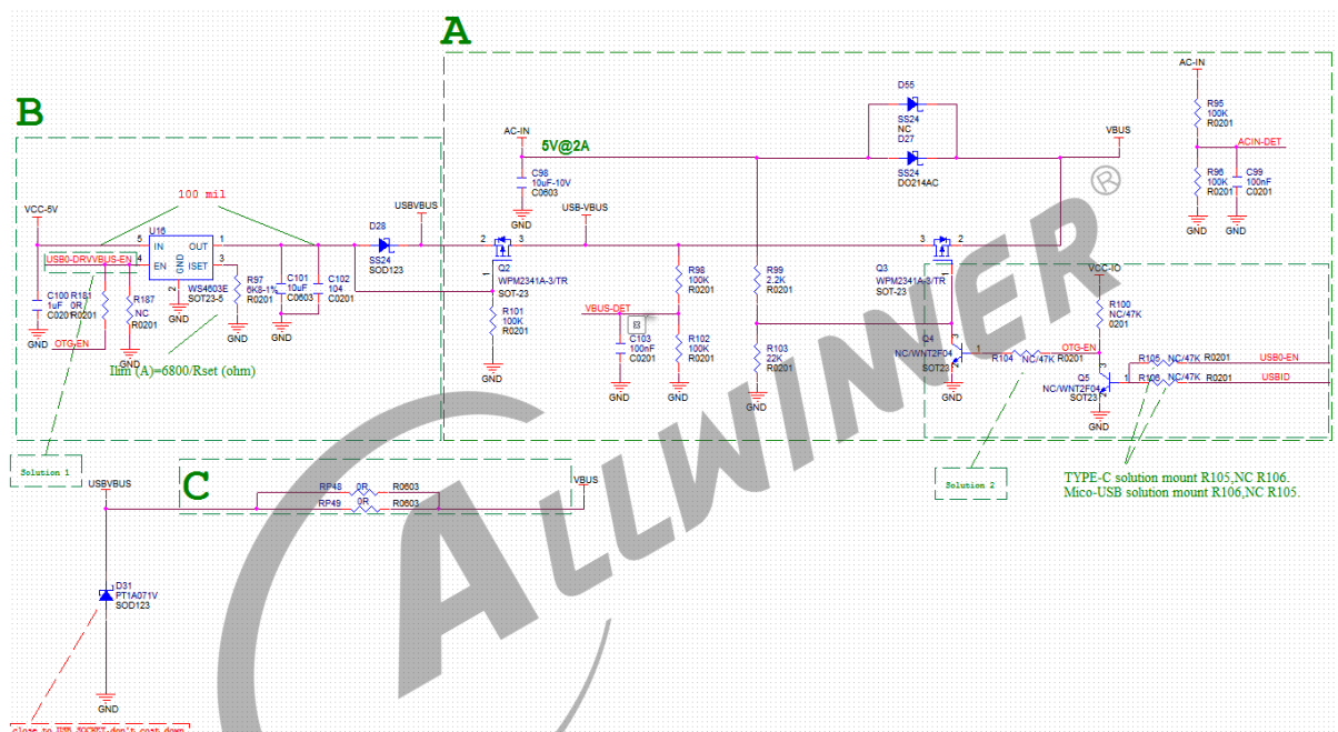
图 7-1: PMIC_ACIN 方案原理图
