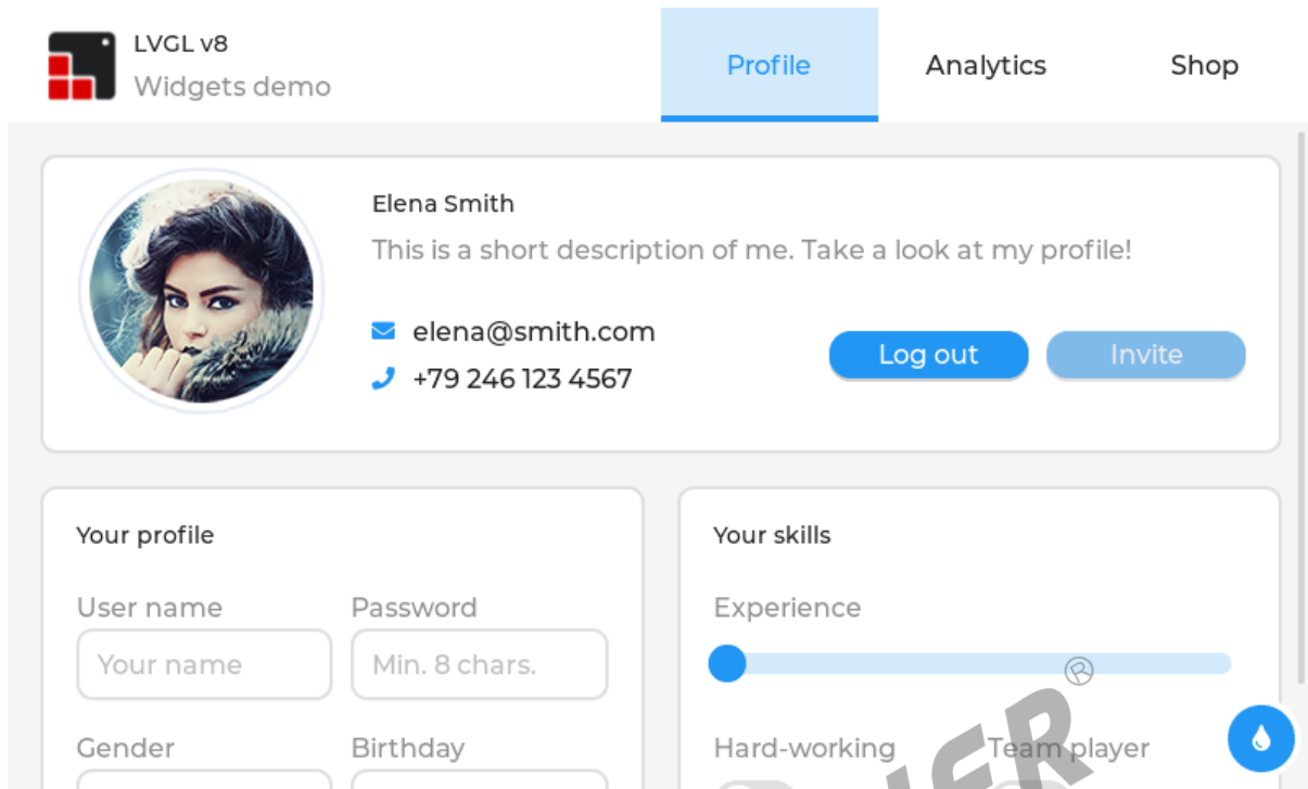
图 8-1: lv_demo_widgets 主页截图
