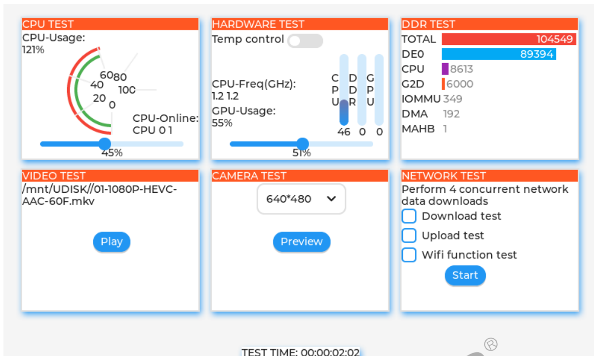
图 8-3: lv_monitor 主页截图
