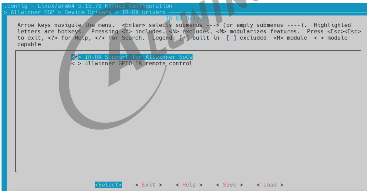
图 4-11: IR-RX_Support
