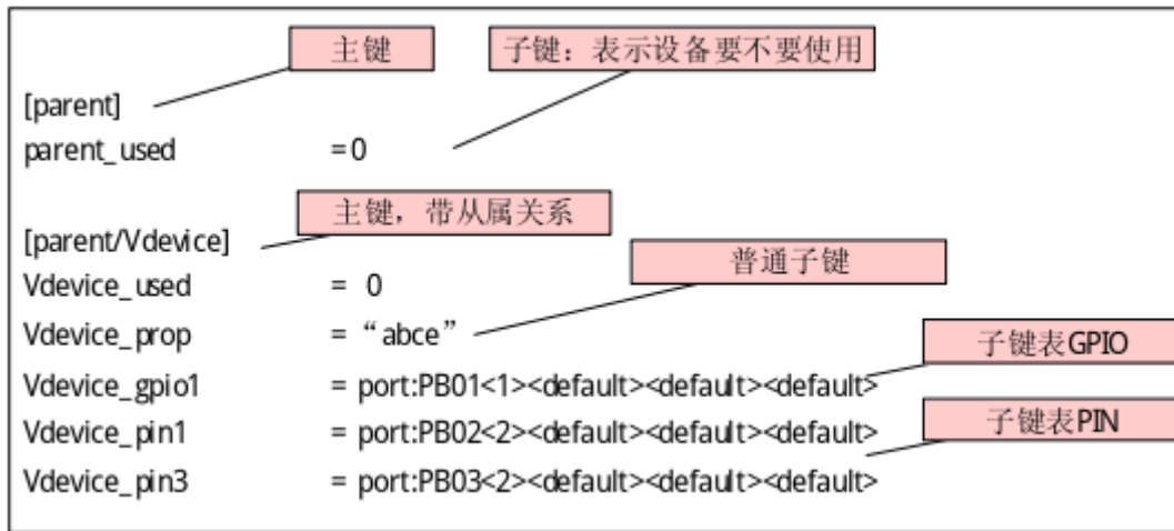
图 5-3: sysconfig 配置
