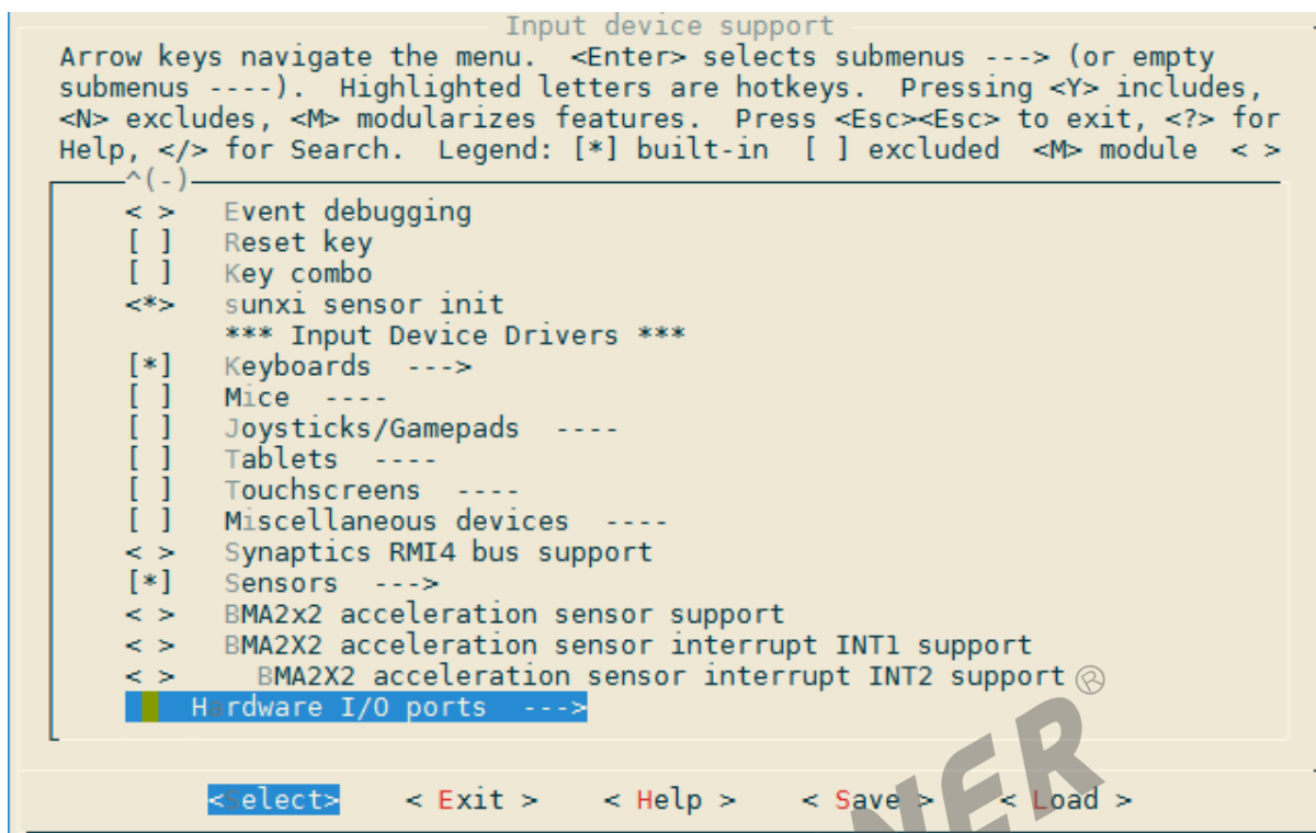
图 2-5: Sensors
