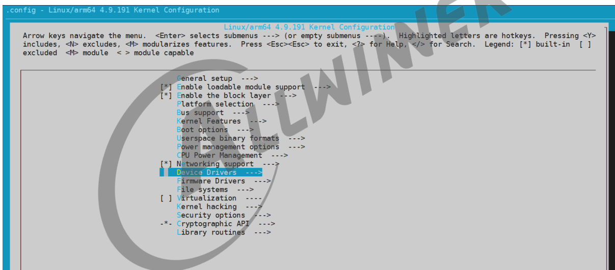
图 3-1: 内核 menuconfig 根菜单
