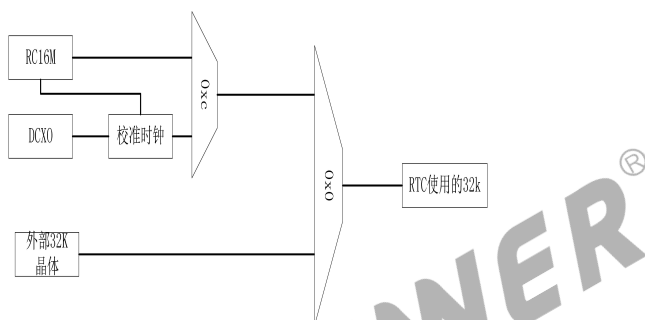
图 6-1: RTC 时钟源
