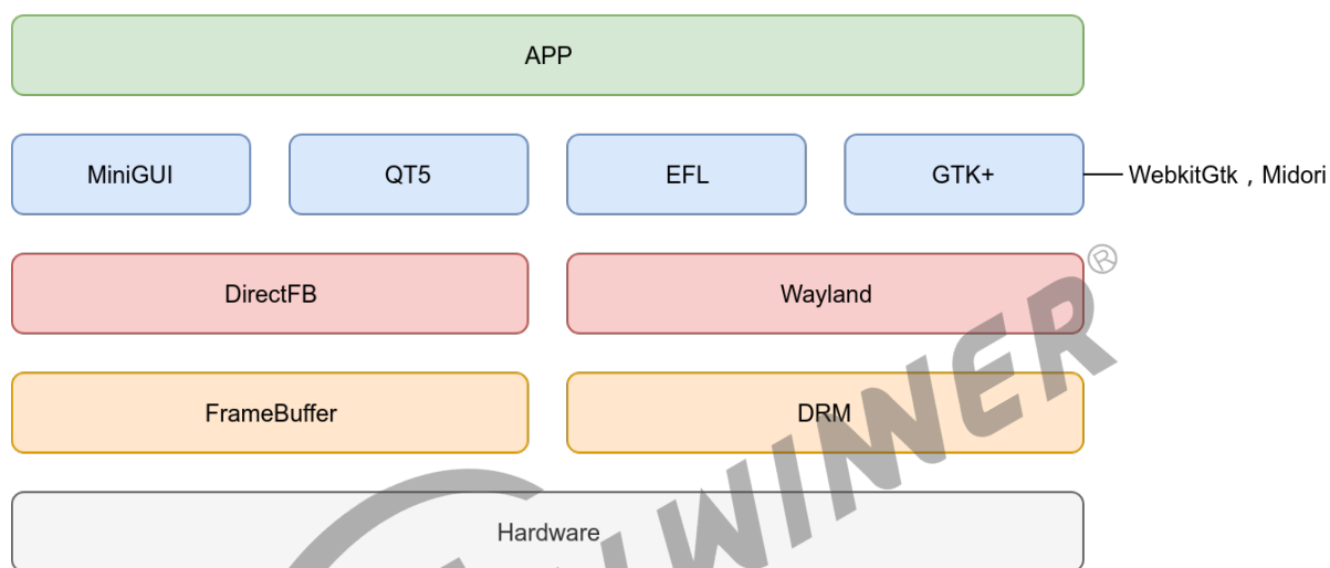
图 1-1: Tina 窗口系统框架
