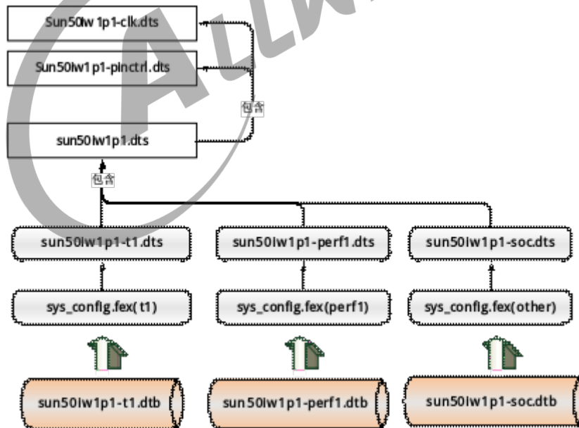
图 5-2: 存在 sysconfig 的配置结构
