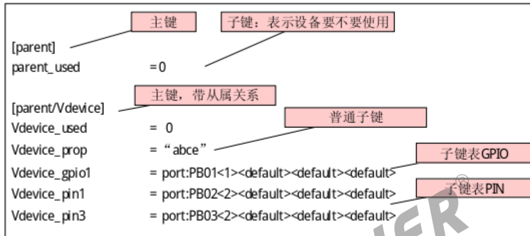
图 5-3: sysconfig 配置
