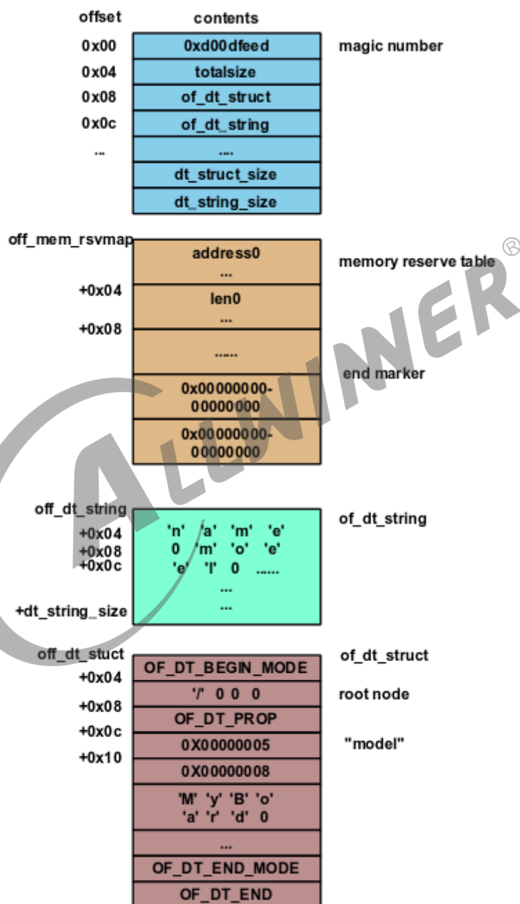
图 4-8: dtb 实例
