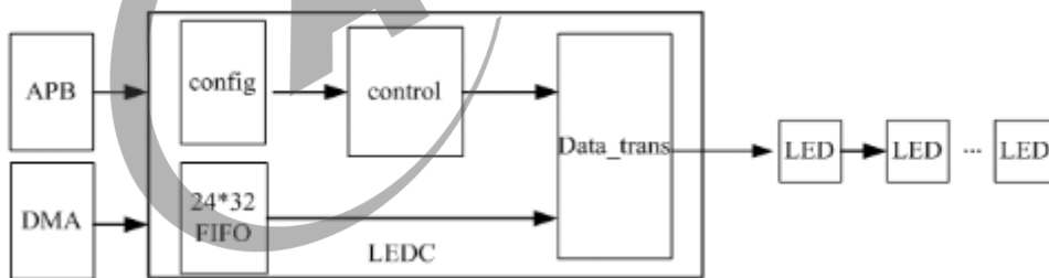
图 2-2: 硬件结构
