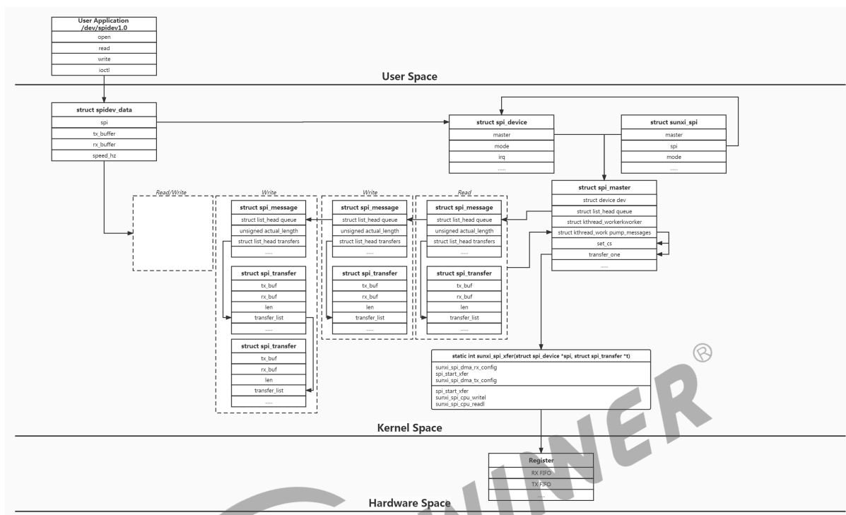
图 4-1: Linux SPI 数据传输流程
