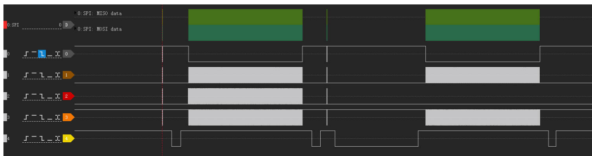
图 5-2: Slave DMA 2048B
