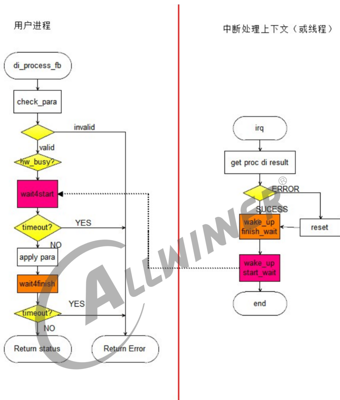
图 5-6: 帧处理流程图
