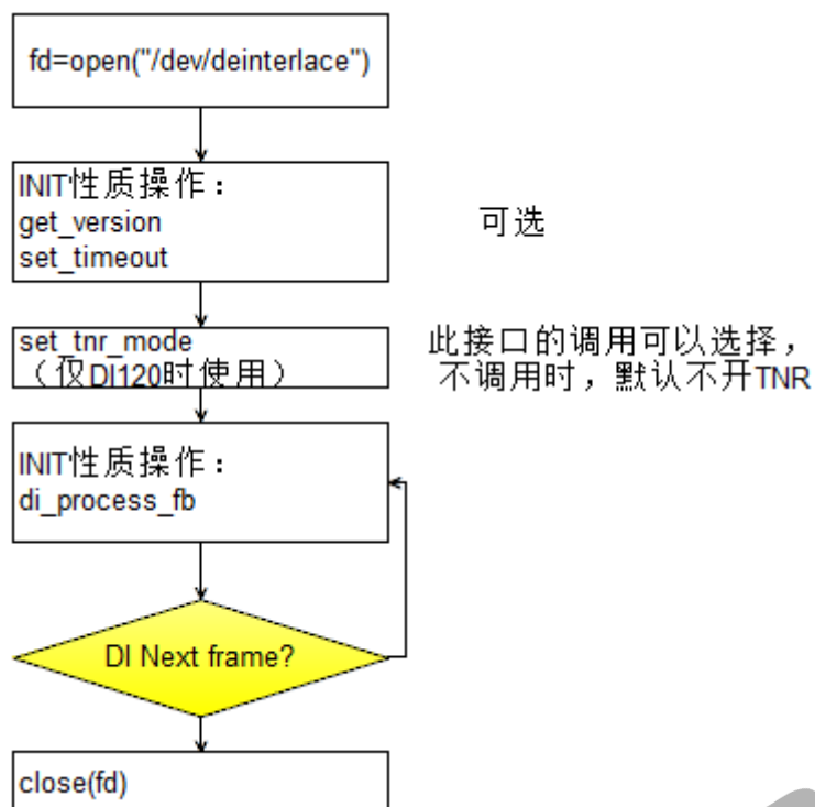
图 5-5: 驱动调用流程图
