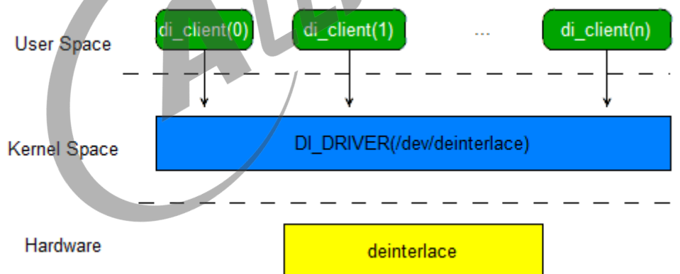
图 5-4: 软件总体架构
