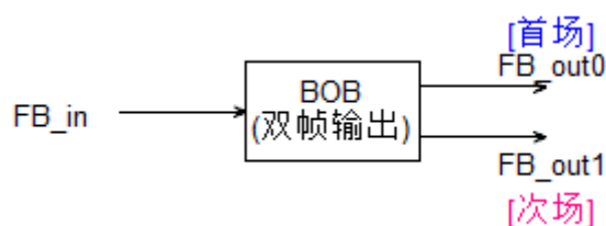
图 5-8: BOB 双帧模式数据流模型
