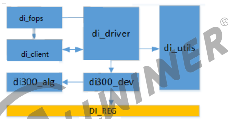
图 4-2: DI 驱动结构
