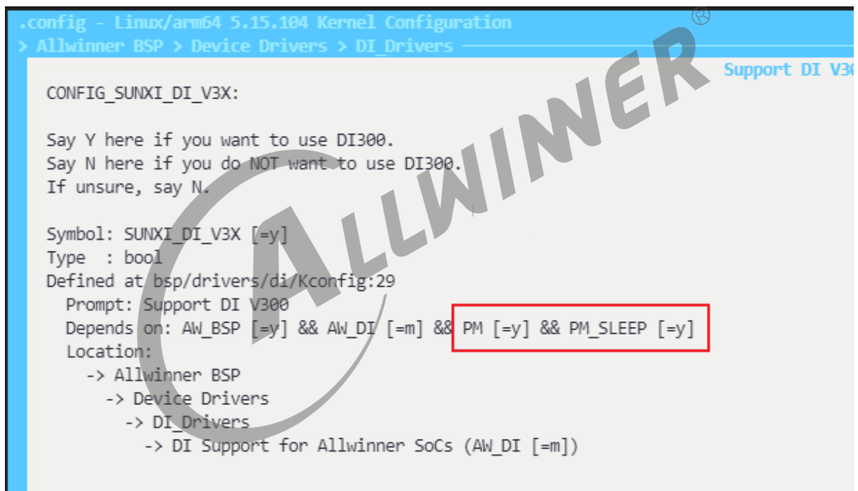
图 2-3: DI300_Help 页面
