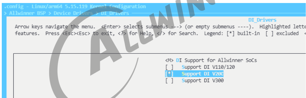
图 4-1: DI menuconfig-5.10
