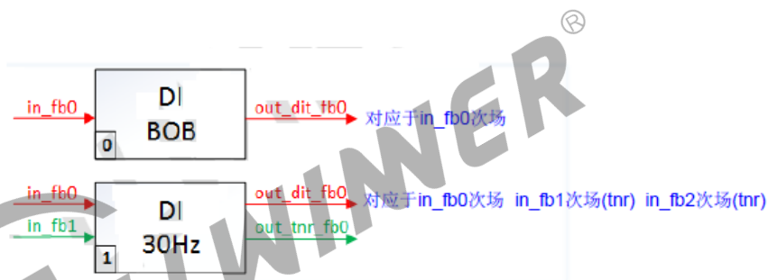
图 2-11: 30Hz 起播流程
