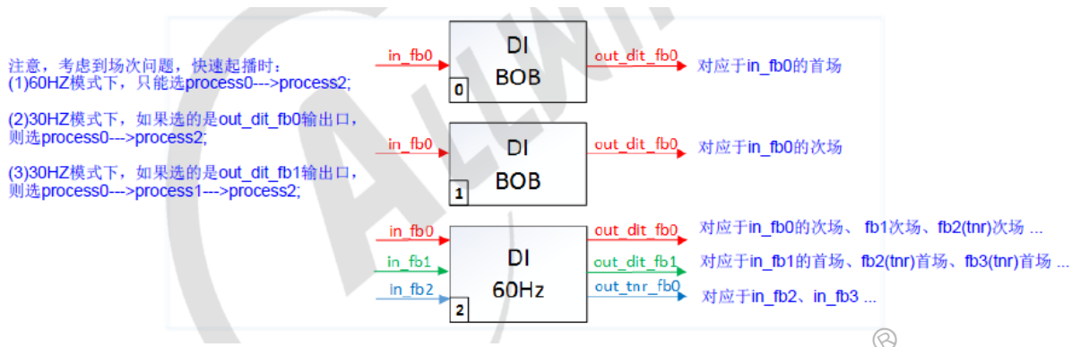
图 2-7: 60 Hz 起播流程
