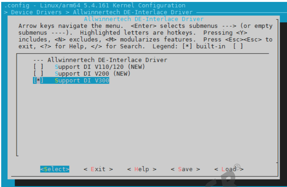
图 2-1: DI menuconfig
