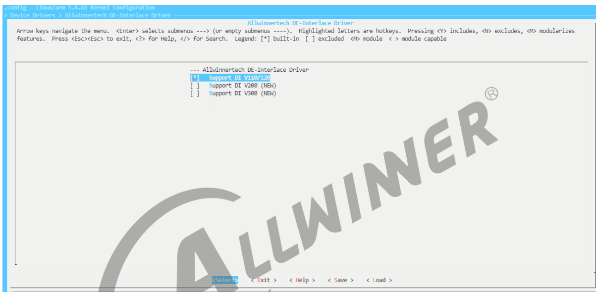
图 5-1: DI menuconfig
