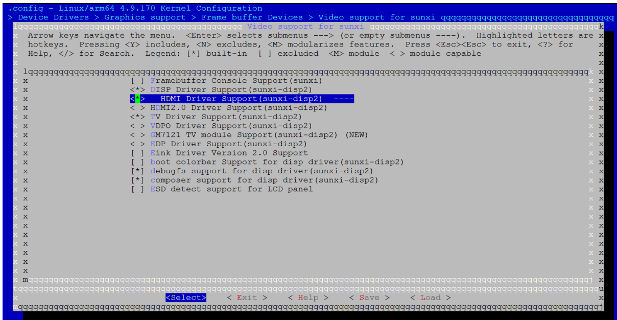
图 2-4: disp2 配置
