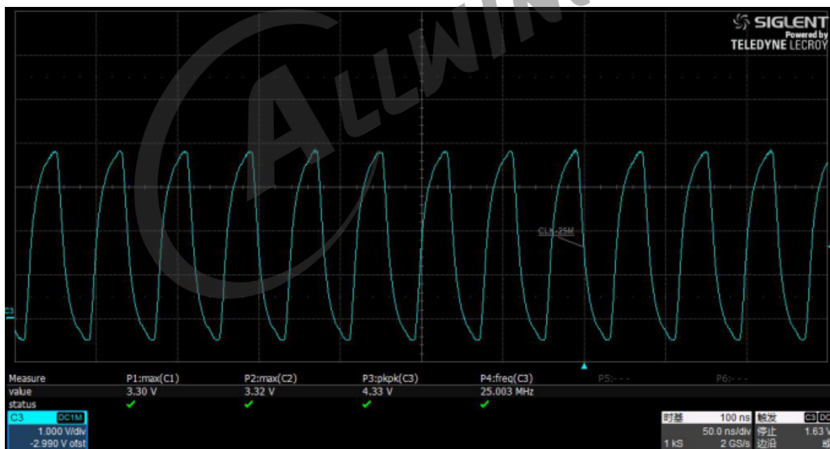
图 6-6: 时钟波形
