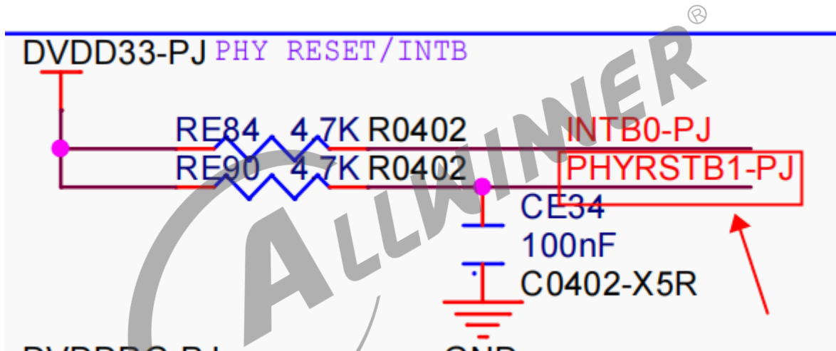
图 6-10: phyrst 原理图
