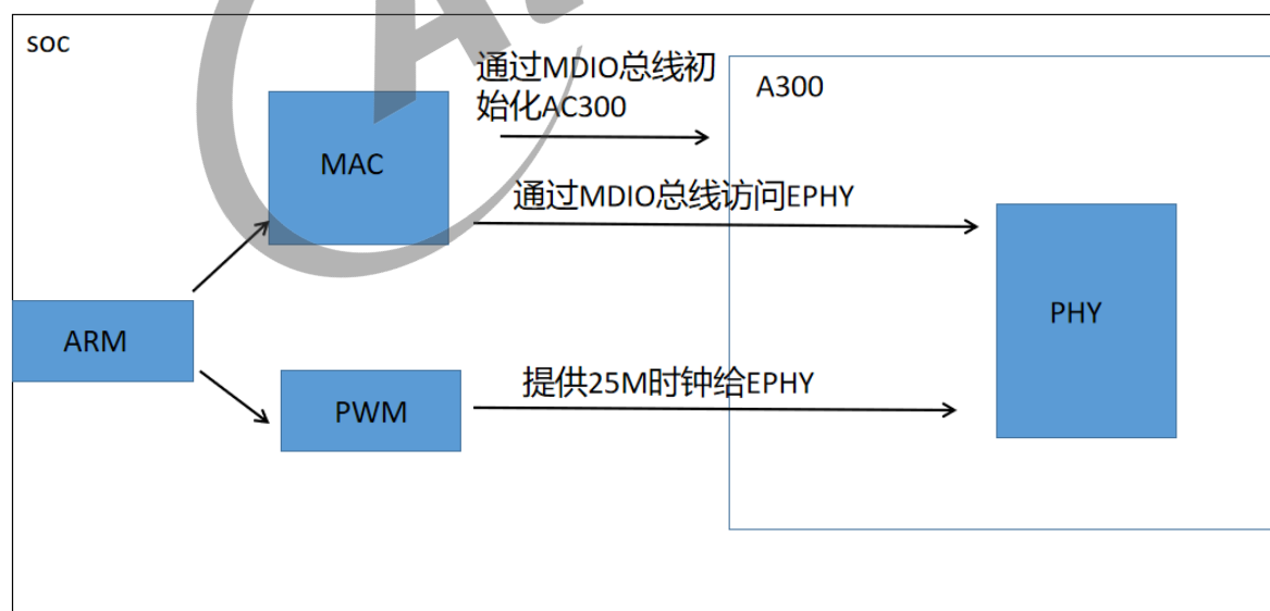
图 3-4: AC300 框图
