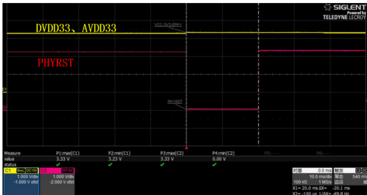
图 6-11: phyrst 波形图
