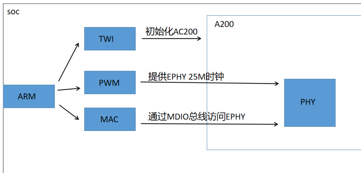
图 3-3: AC200 框图
