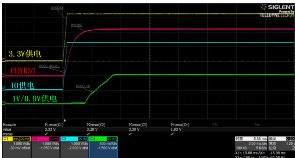
图 6-8: 上电时序
