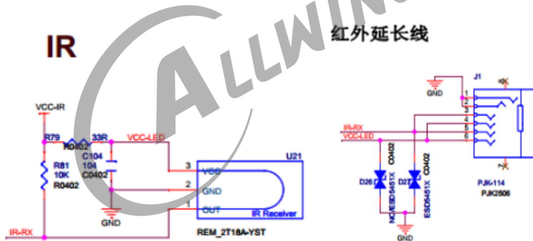
图 2-1: IR-RX 模块
