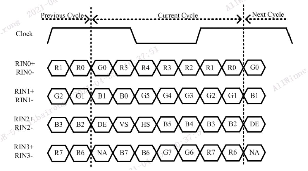
图 14-1: lvds mode jedia
