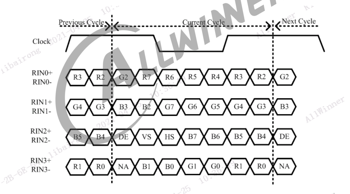
图 14-2: lvds mode ns
