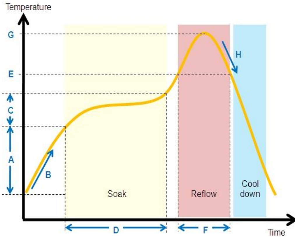
图 2-2 焊接温度曲线
