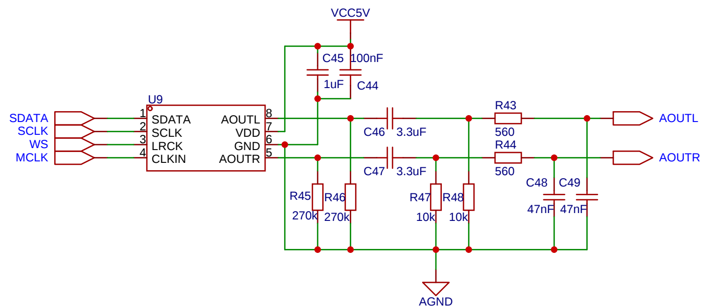
立体声DA转换器
