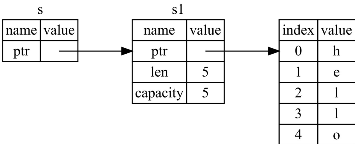
图 4-5： &String s 指向 String s1 示意图
