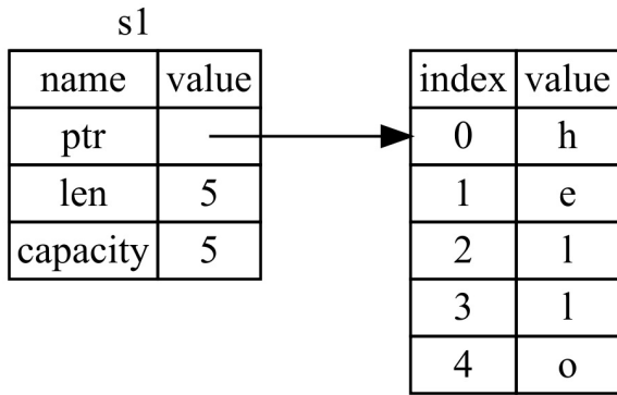
图 4-1：将值 "hello" 绑定给 s1 的 String 在内存中的表现形式
