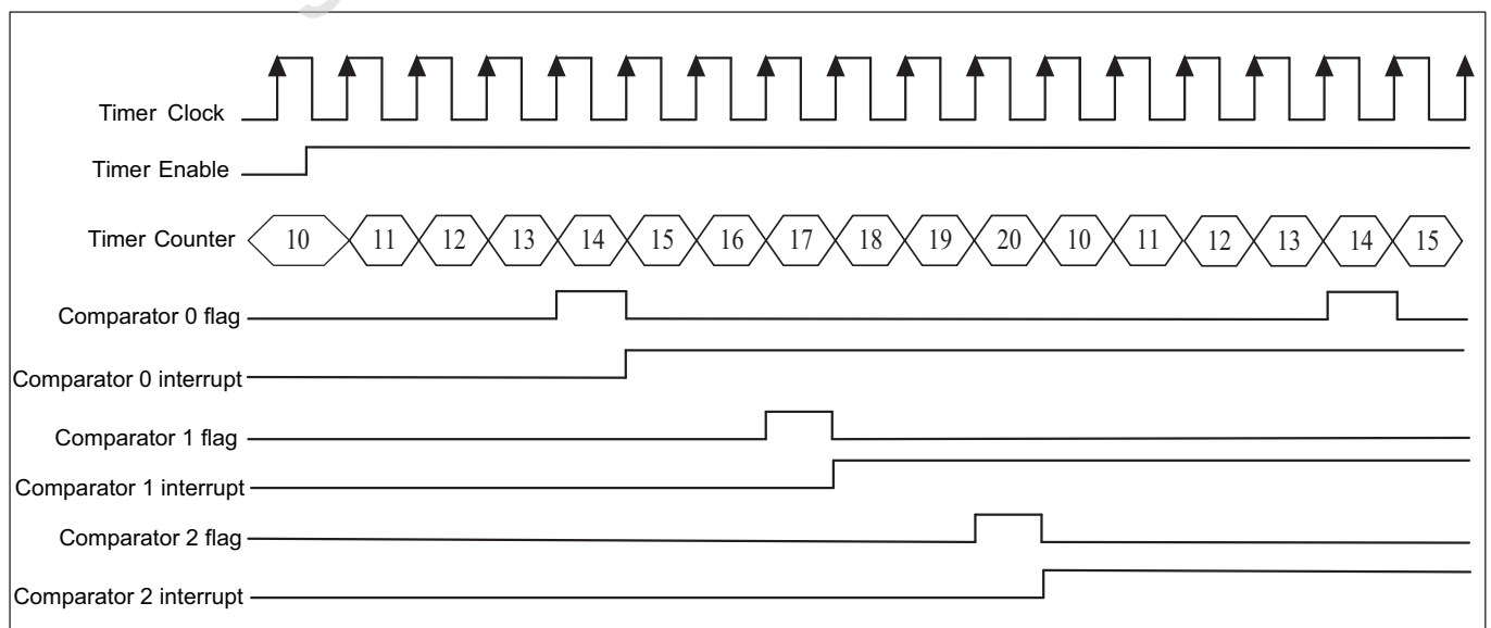
Fig. 13.3: Timer Preload
