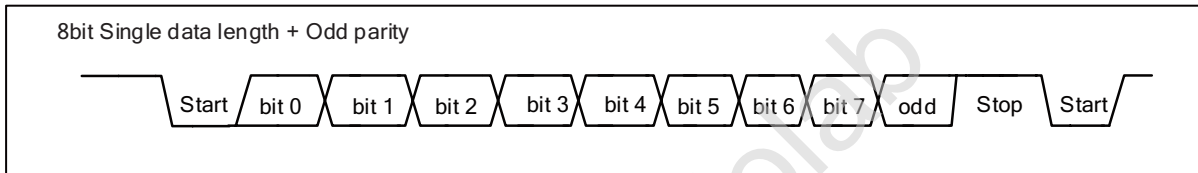
Fig. 10.1: UART data
