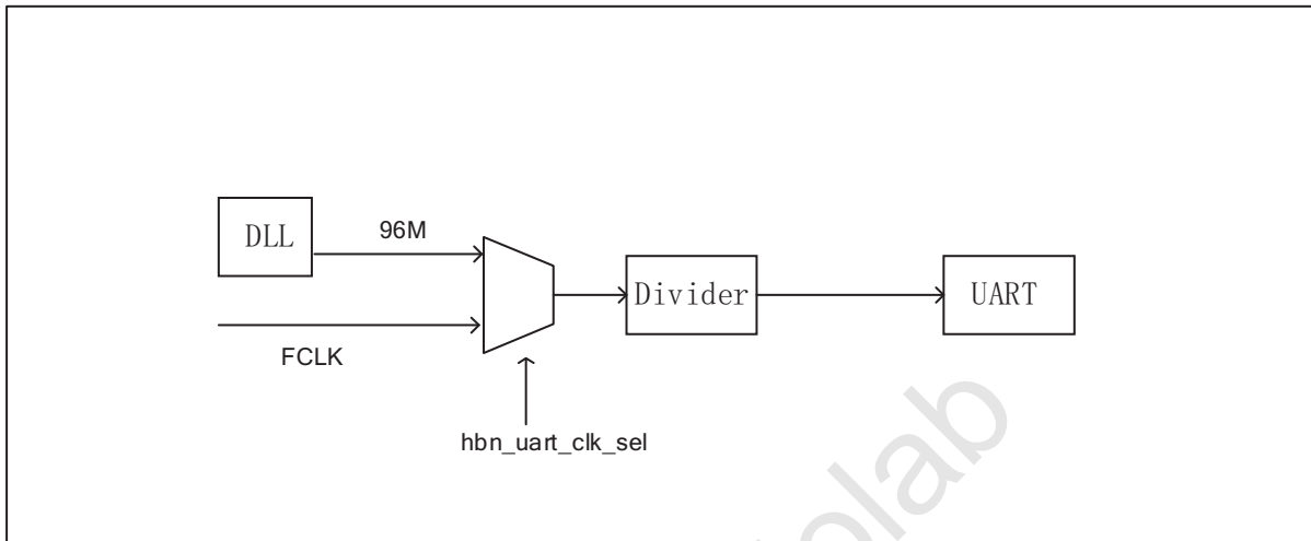
Fig. 10.2: UART clock
